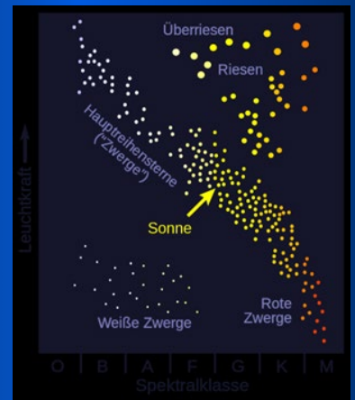
Schwarzschild und Schwarzes Loch (© AIP); Karl Schwarzschild (1873-1916) und Ejnar Hertzsprung (1873-1967); Hertzsprung-Russell-Diagramm (CC3, sparse-Rursus)
